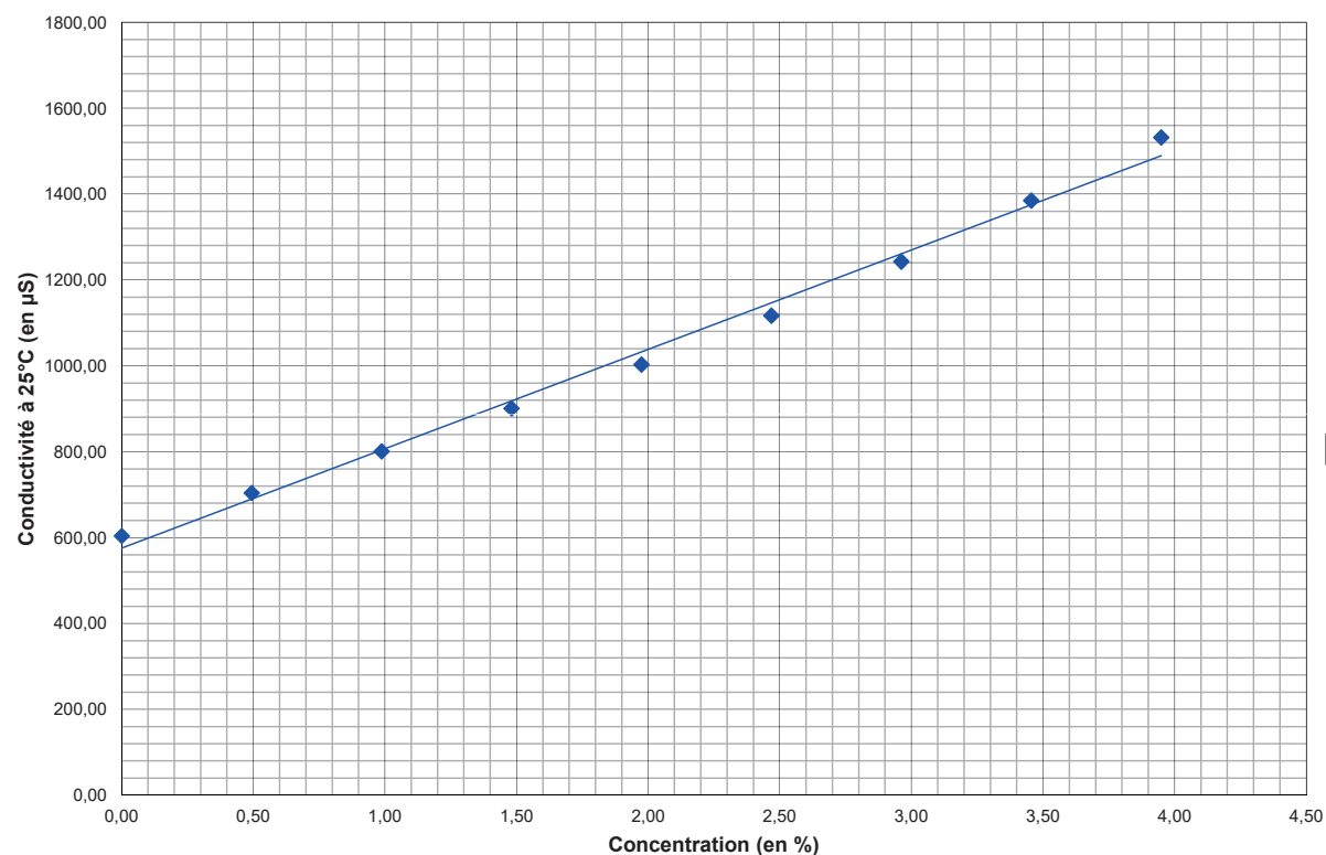
Courbe de conductivité à 25°C du DETERQUAT DNA- V2 Courbe réalisée avec une eau de dureté = 18°f avec le conductimètre WTW Cond 3110
